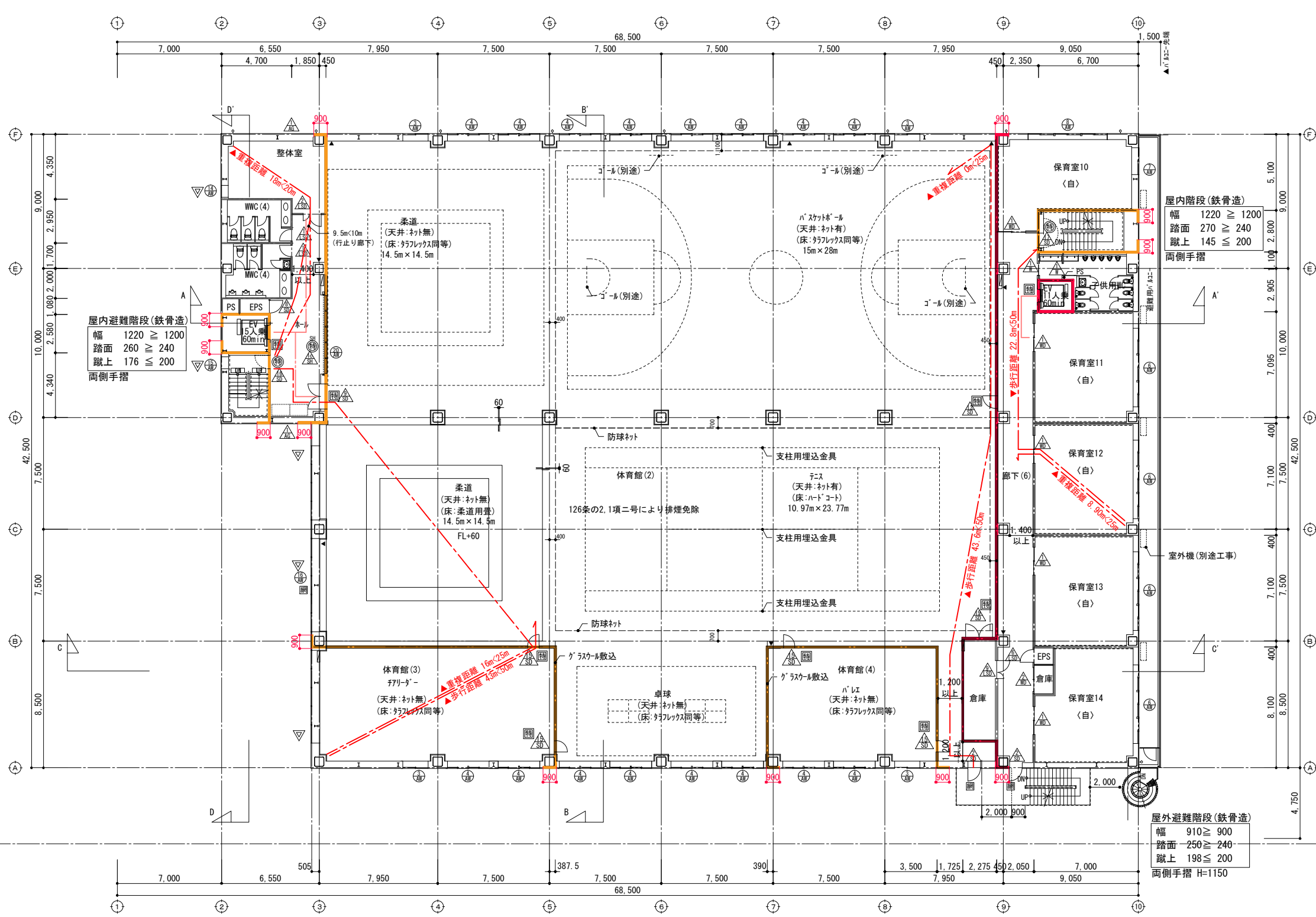
3階平面図 A1:S=1/150 A3:S=1/300
